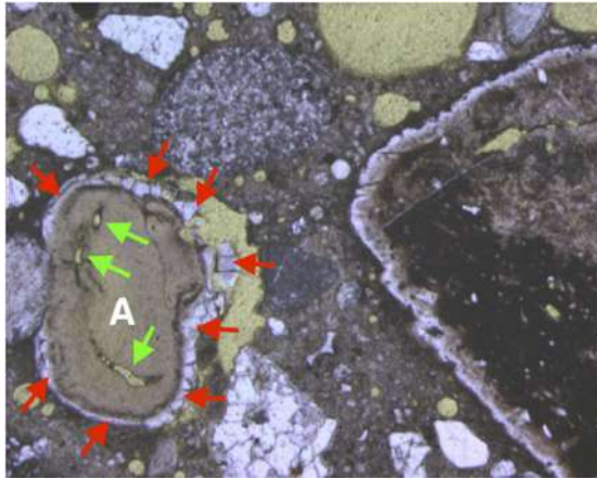
Şekil 16. Agregada etrafında ASR jeli oluşumu (kırmızı oklar)
