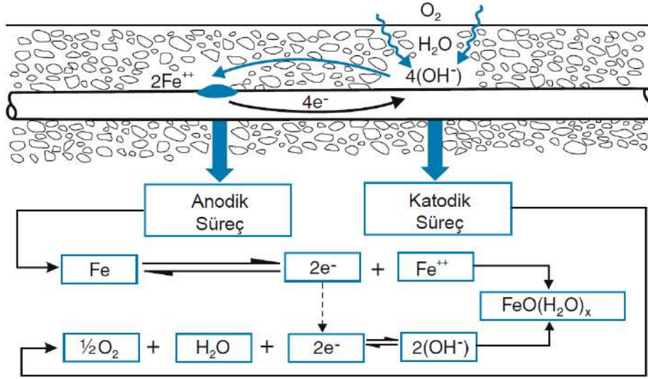
Şekil 10. Çelik donatıda korozyon oluşumu
